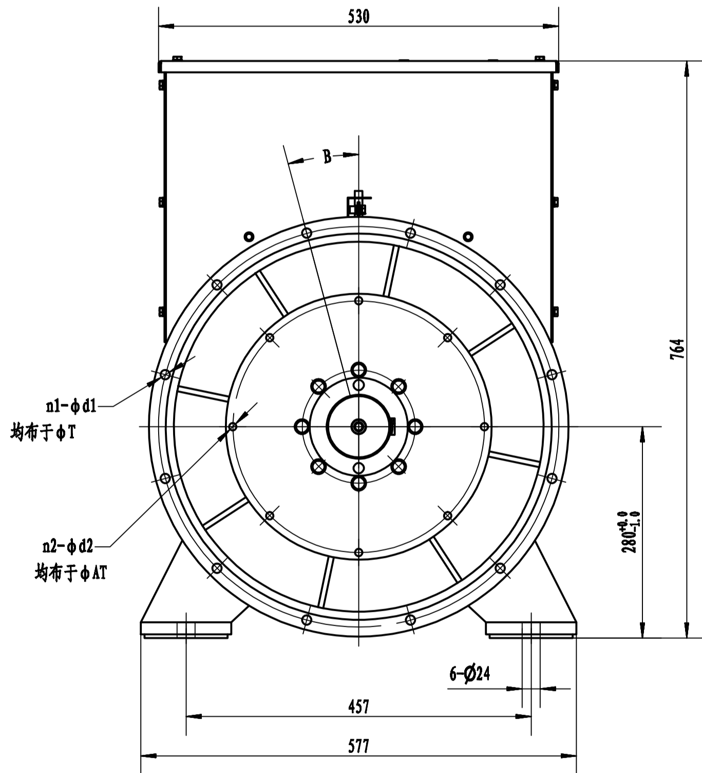
过渡连接尺寸 (FLANGE DIMENSION)
